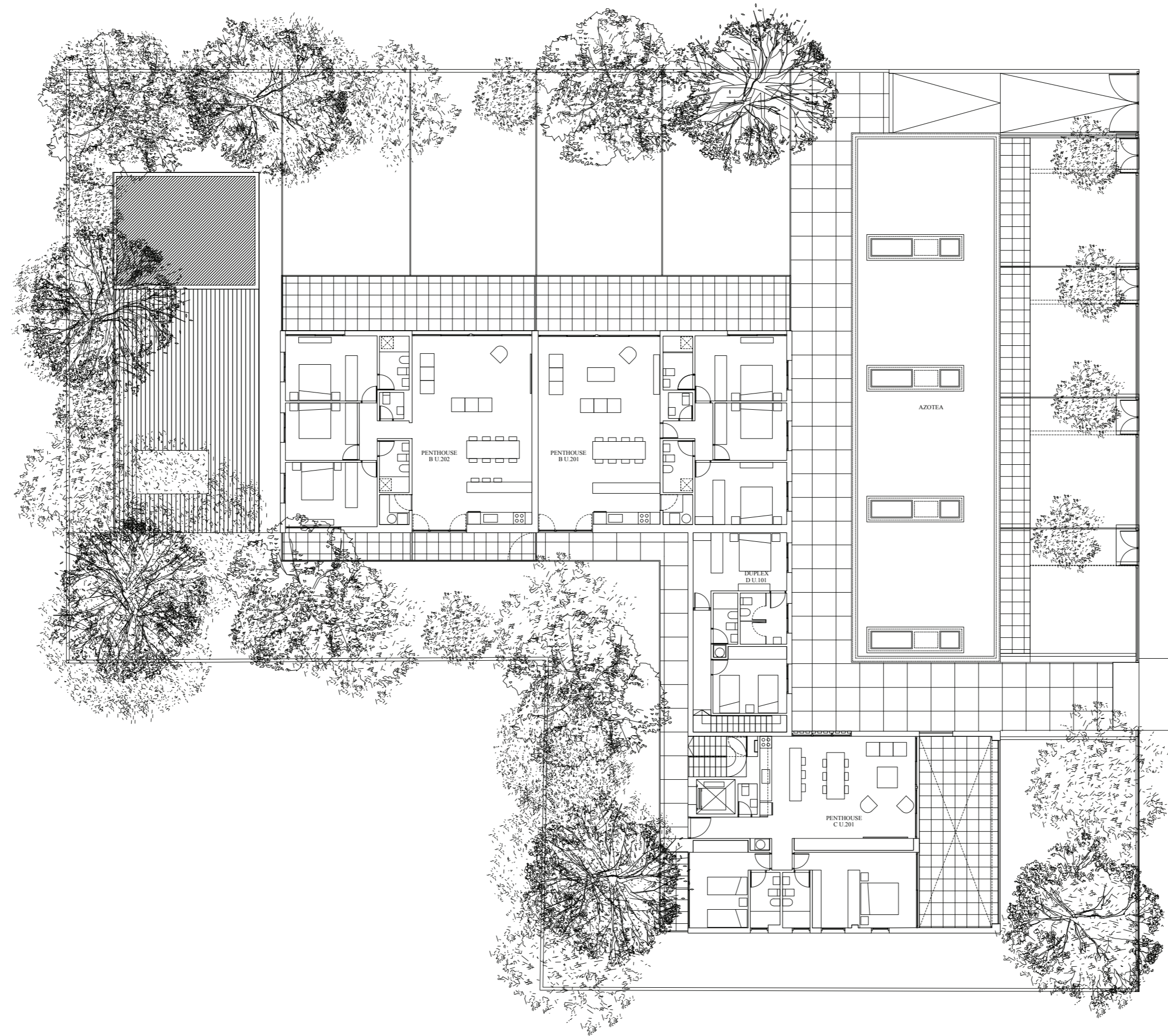
PLANTA NIVEL 2
